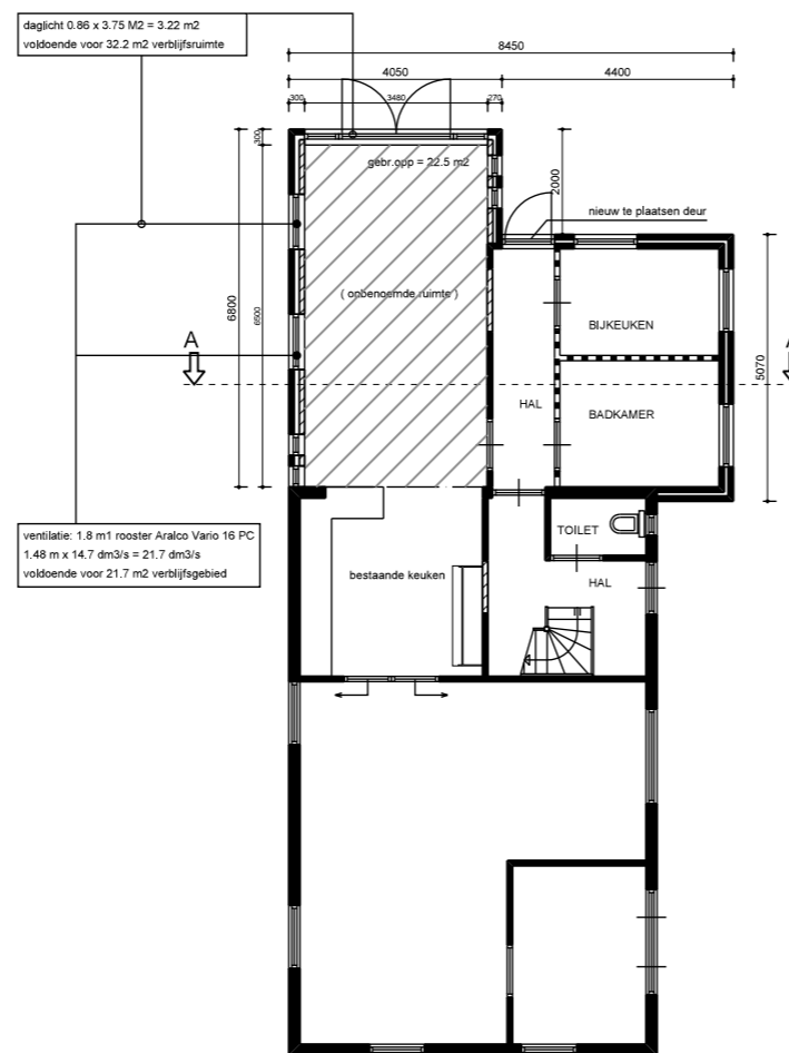
plattegrond nieuw
