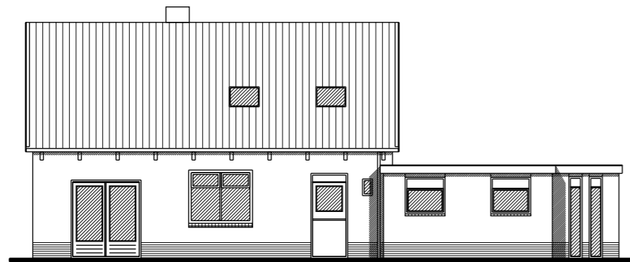
rechter zijgevel nieuw
