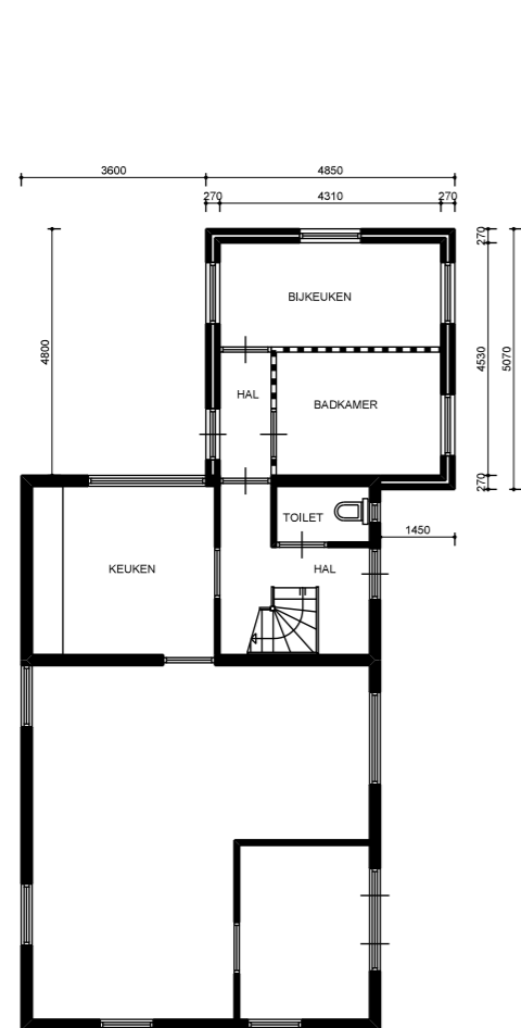
plattegrond bestaand
