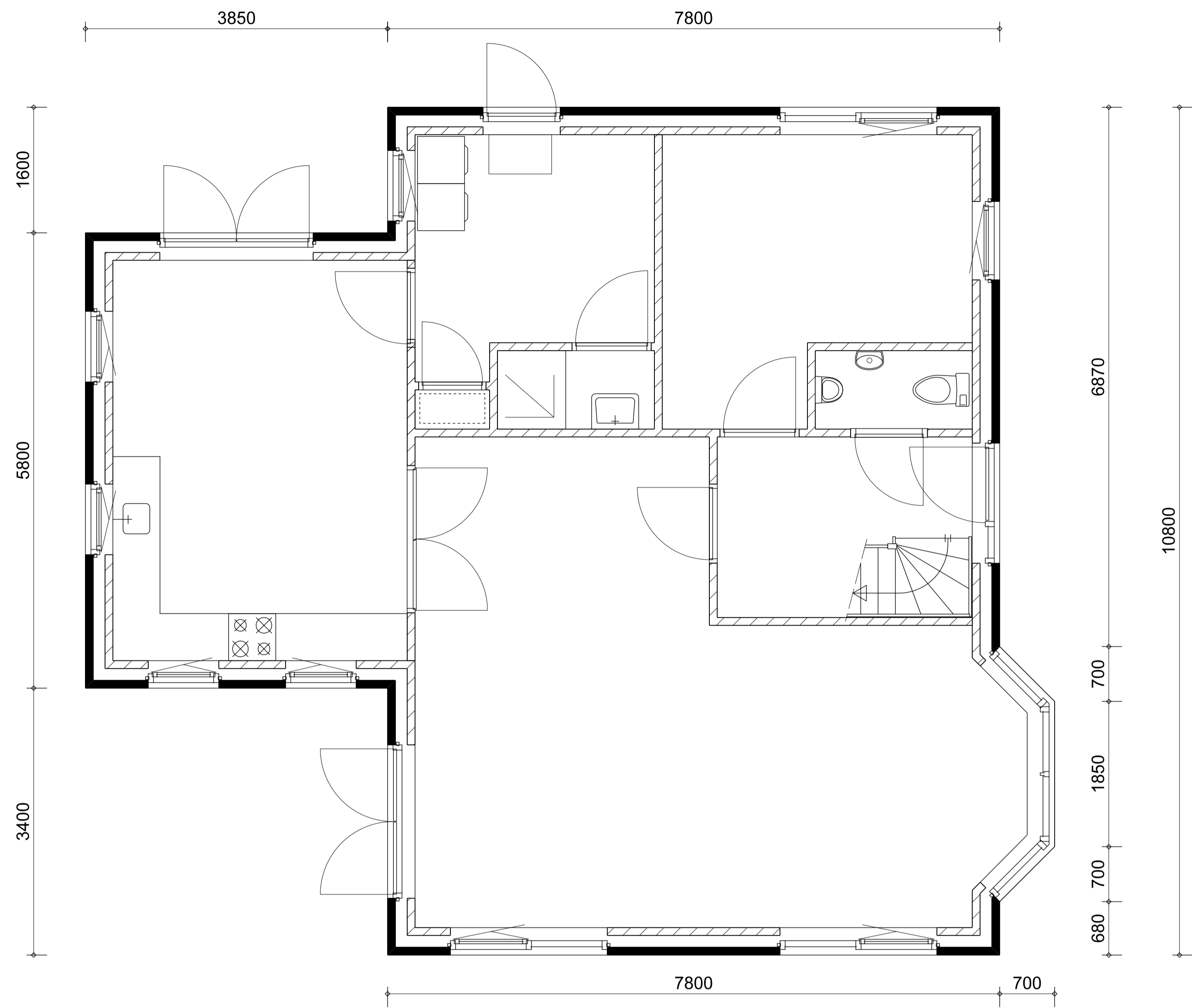
BEGANE GROND
