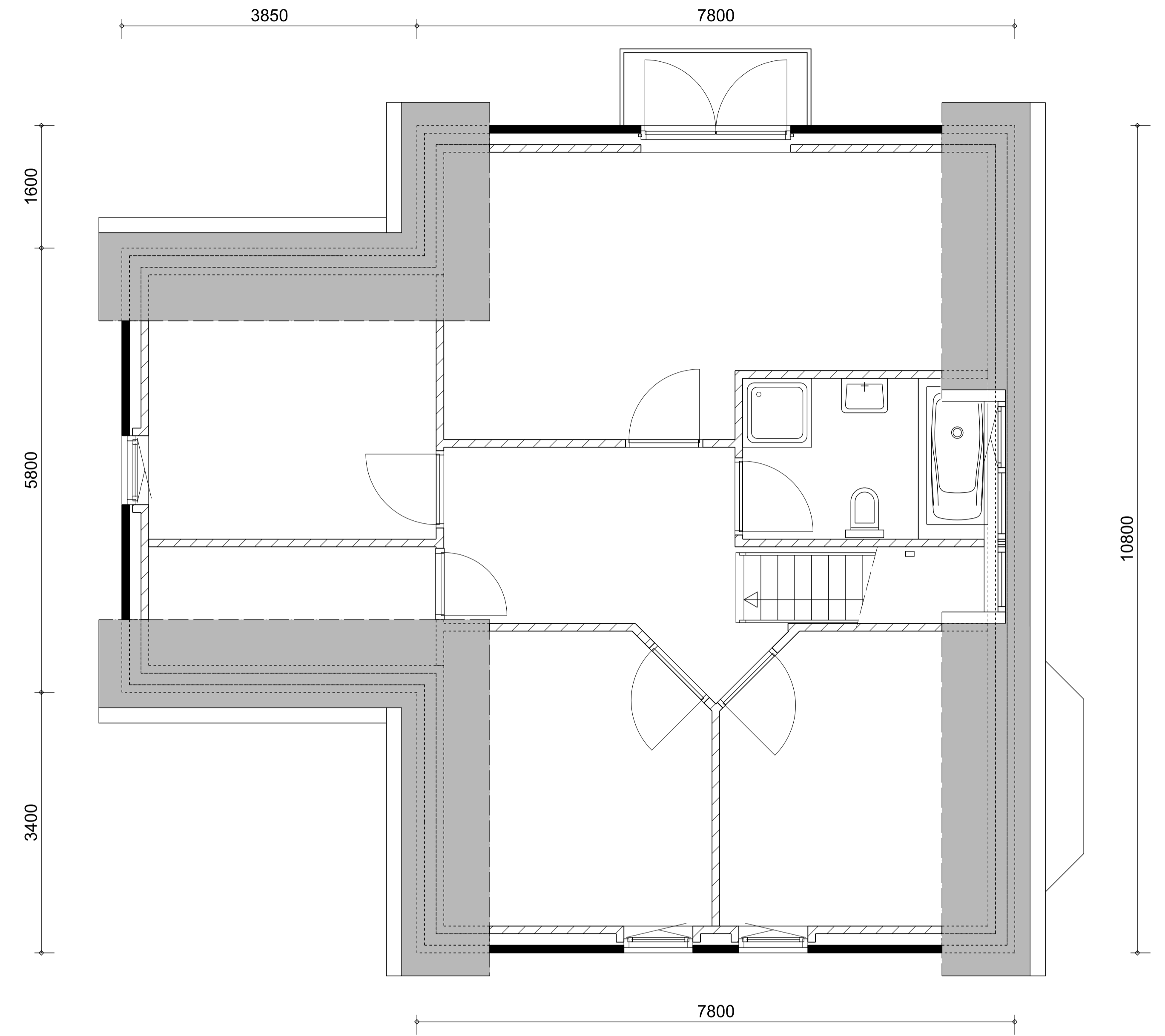
1e VERDIEPING
