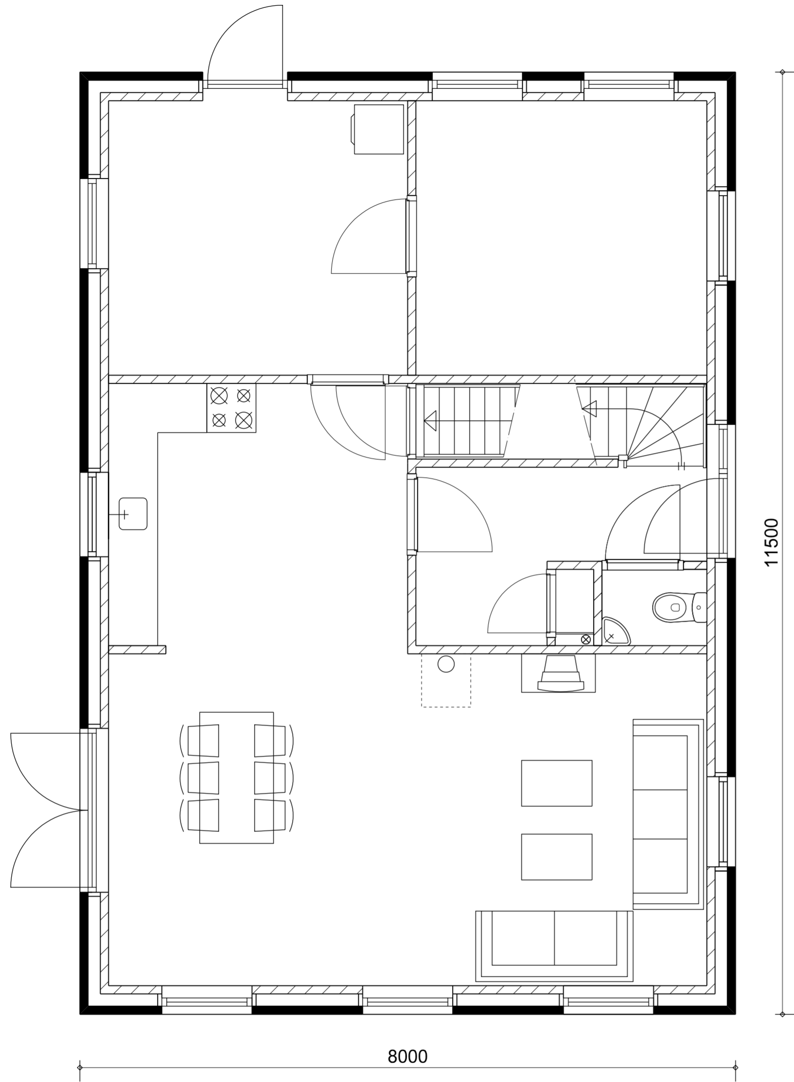
BEGANE GROND
