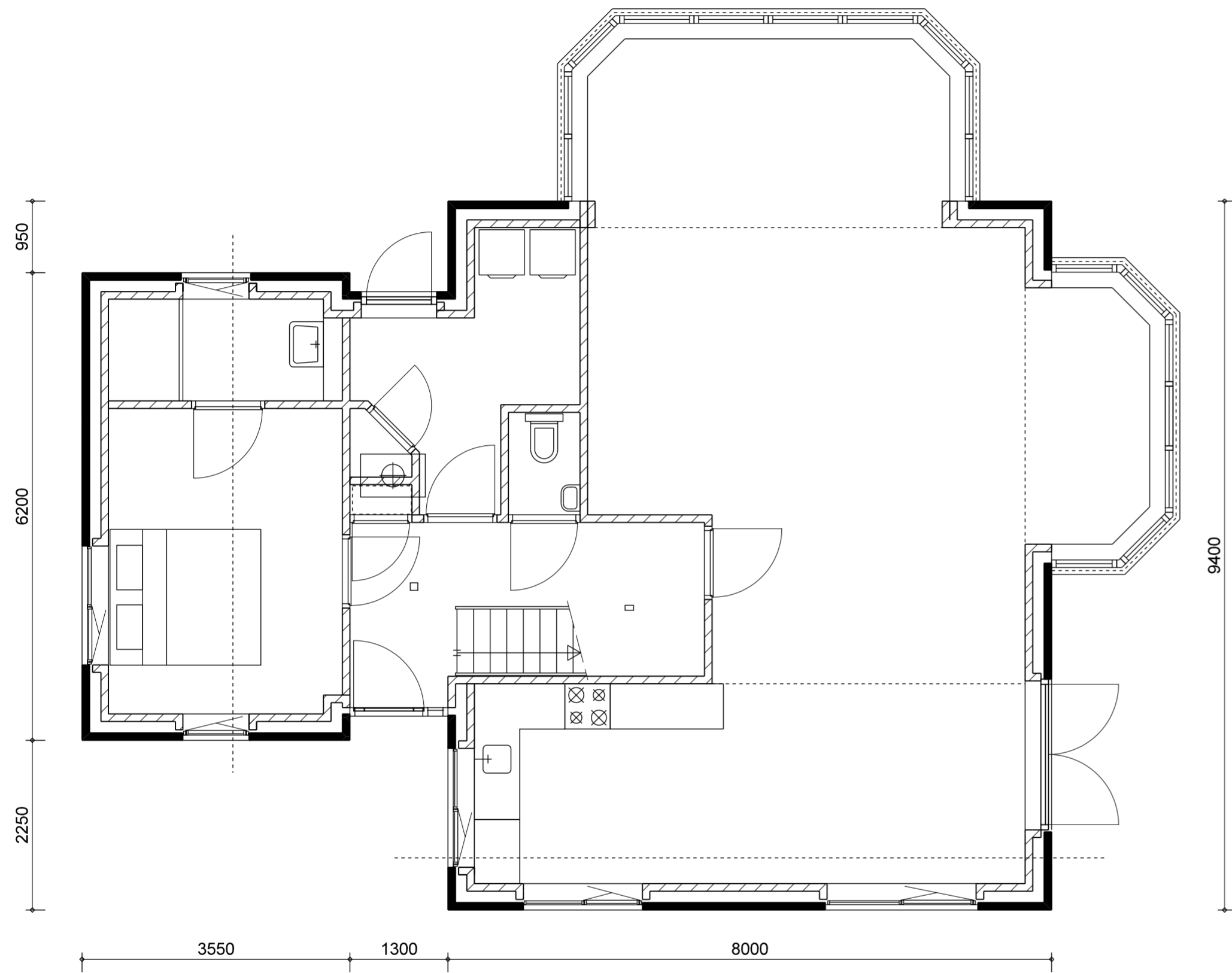
BEGANE GROND
