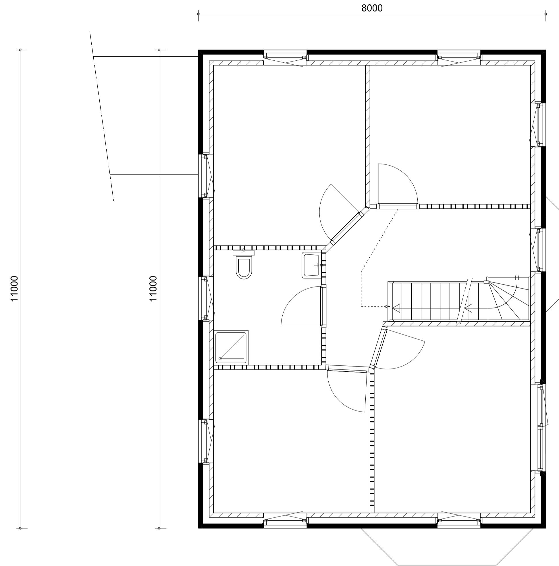
1E VERDIEPING
